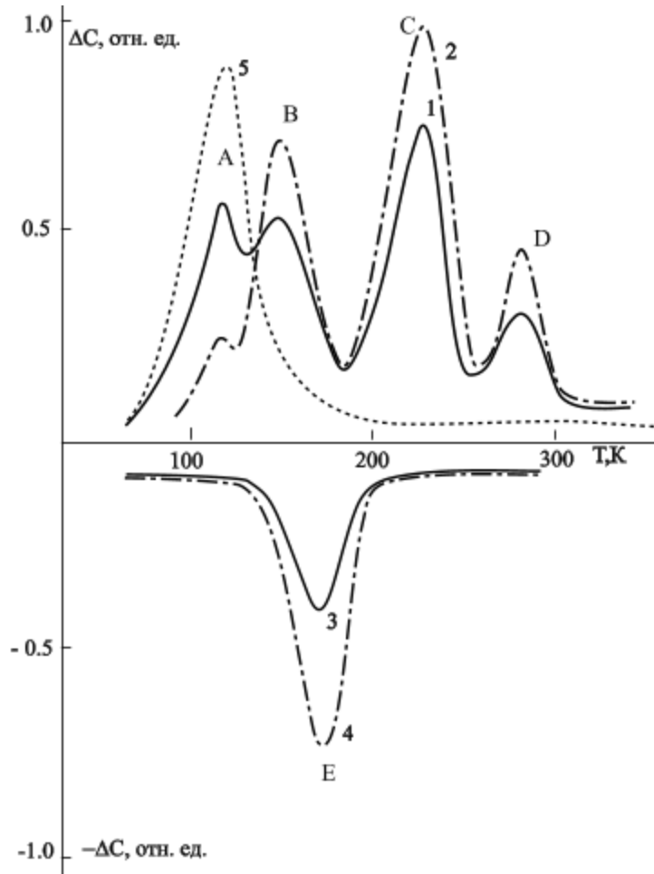
Рис. 1. Типичные спектры DLTS образцов n\text{-Si}\langle\text{Co}\rangle (1), n\text{-Si}\langle\text{Gd,Co}\rangle (2), p\text{-Si}\langle\text{Co}\rangle (3), p\text{-Si}\langle\text{Gd,Co}\rangle (4) и контрольного образца (5)
