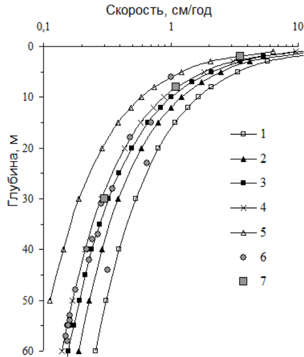
Рис. 1. Модель динамики верхней границы многолетнемерзлых пород исследуемых районов арктического шельфа в поле отрицательных температур. Скорость диффузии солей с концентрацией на подвижной границе фазового перехода: 1 – 1 ‰, 2 – 2 ‰, 3 – 3 ‰, 4 – 4 ‰, 5 – 10 ‰. Скорость деградации мерзлоты: 6 – по результатам моделирования, 7 – оцененная по данным бурения на шельфе моря Лаптевых [8]
