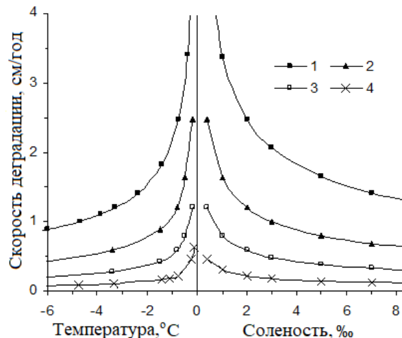
Рис. 2. Изменения скорости деградации твердомерзлых пород верхнего горизонта на шельфе Восточно-Сибирского моря в зависимости от температуры замерзания и солёности поровых вод на границе фазовых переходов, залегающей на глубинах: 1 – 5 м, 2 – 10 м, 3 – 20 м, 4 – 50 м от поверхности дна
