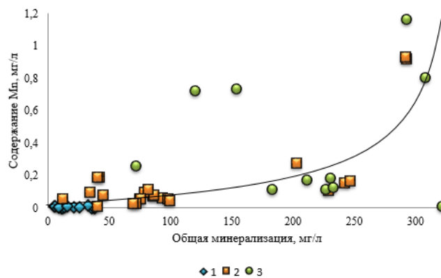
Рис. 5. Зависимость содержания железа общего (а) и марганца (б) от общей минерализации 1 – снег, 2 – поверхностные воды, 3 – подземные воды
