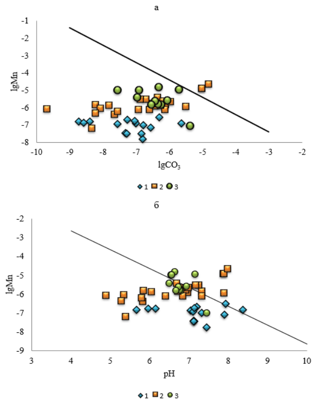
Рис. 6. Степень насыщенности природных вод ХМАО по родохрозиту (а) и по пирохроиту (б) 1 – снег, 2 – поверхностные воды, 3 – подземные воды
