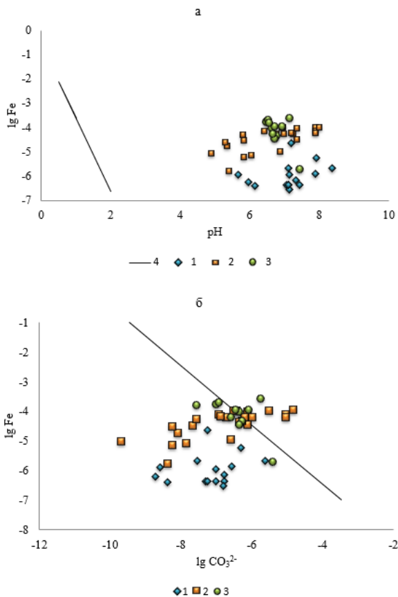
Рис. 4. Степень насыщенности природных вод ХМАО по гетиту (а) и сидериту (б). 1 – снег, 2 – поверхностные воды, 3 – подземные воды
