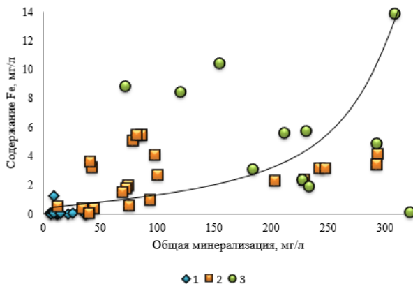
Рис. 3. Зависимость содержания железа общего от общей минерализации 1 – снег, 2 – поверхностные воды, 3 – подземные воды
