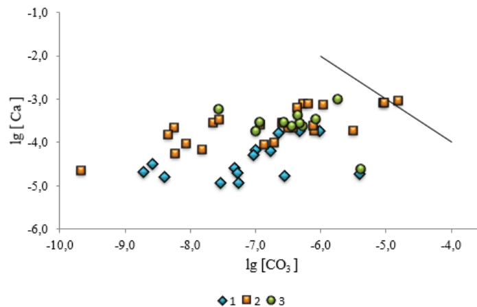
Рис. 1. Степень насыщенности природных вод на территории ХМАО относительно \text{CaCO}_3 1 – снег, 2 – поверхностные воды, 3 – подземные воды
