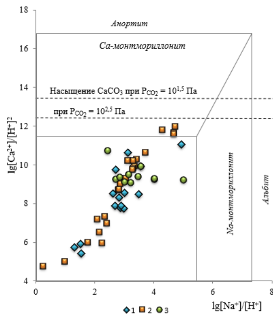
Рис. 2. Диаграмма равновесия в системе вода – алюмосиликаты в природных водах ХМАО 1 – снег, 2 – поверхностные воды, 3 – подземные воды
