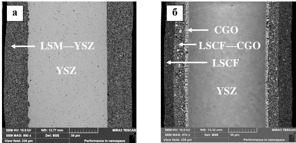
Рис. 1. Микрофотография сечения: а – LSM – YSZ / YSZ / LSM – YSZ; б) – LSCF – CGO / CGO / YSZ / CGO / LSCF – CGO
